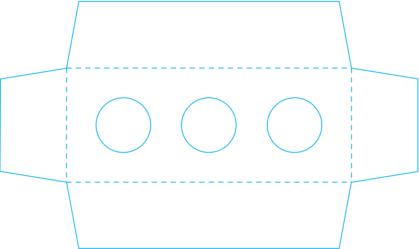
400g灰底白板纸120×48×28mm 展开尺寸176×104mm
