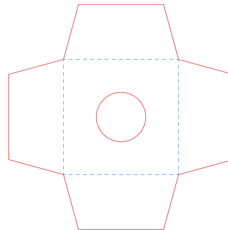
401020740-00615 400g灰底白板纸63×63×φ27×30mm 展开尺寸：123×123mm
